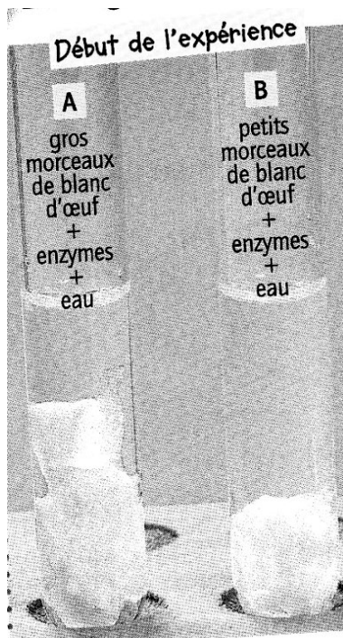
Photographies des expériences réalisées et des résultats obtenus 2 heures plus tard à 37°C
