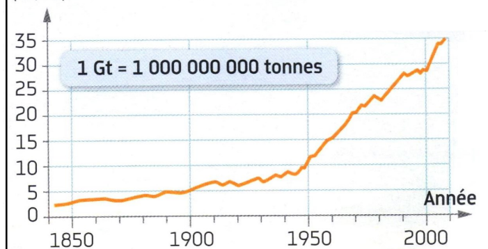
Doc. 3 : Graphique de la quantité de CO 2 libérée par les activités humaines depuis 1850.
