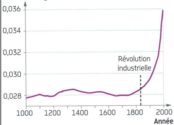
Doc. 2 : Graphique de la teneur en CO 2 dans l'atmosphère depuis l'an 1000
