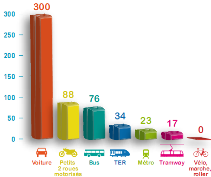
EMISSION DE GAZ À EFFET DE SERRE PAR MODE DE TRANSPORT (TRANSPORT DES PERSONNES) EN GRAMMES ÉQUIVALENT CO 2 PAR KM
