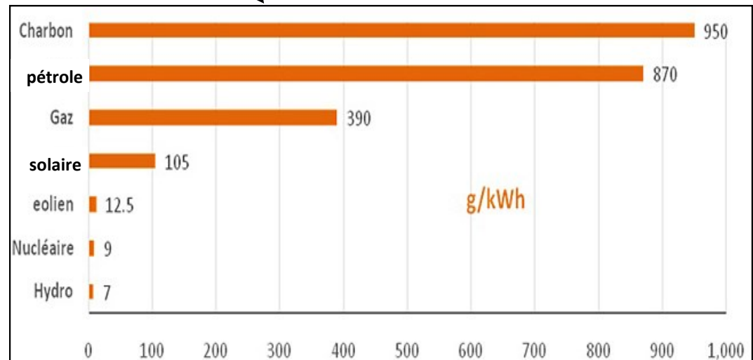
Graphique des émissions de CO 2 par moyen de production d'électricité (en grammes de CO 2 par kilowattheure d'électricité)
