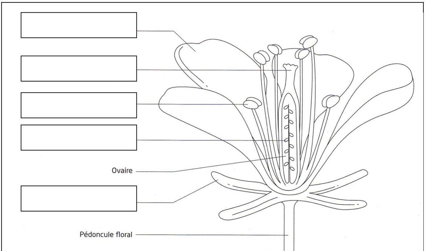
Titre : Schéma d'une coupe de fleur (fleur coupée en deux dans la longueur)
